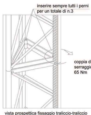
vista prospettica fissaggio traliccio-traliccio
