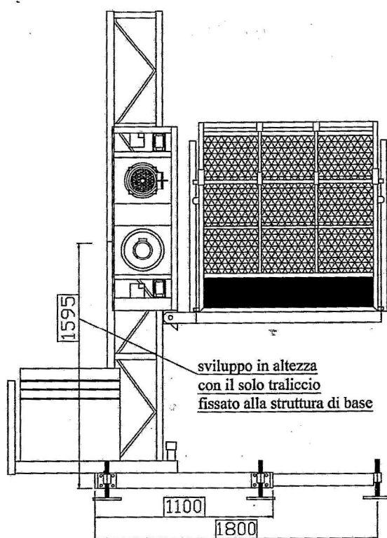
PROSPETTO LATERALE
